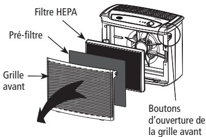
Figure 1 - Modèles 30117, 30119 et 30145
